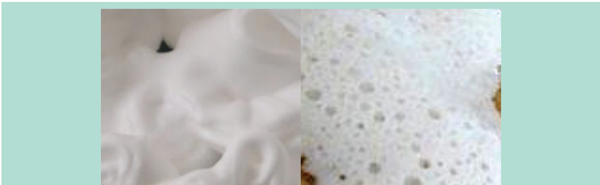
FIGURE 9 : Aspect d'une mousse sèche : ratio < 5 % (à gauche). Aspect d'une mousse humide : ratio > 5 % et < 36 % (à droite).
